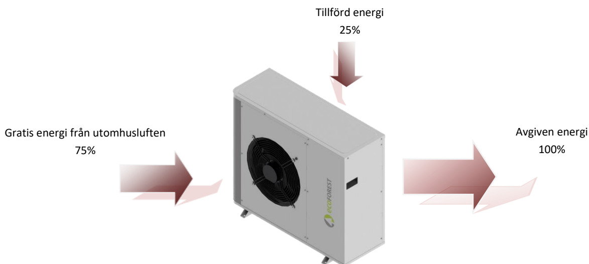
Bild 2.2. En arotermisk värmepumps drift under normala förhållanden.
