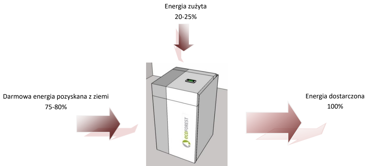
Rysunek 2.1. Działanie geotermalnej pompy ciepła w warunkach normalnych.
