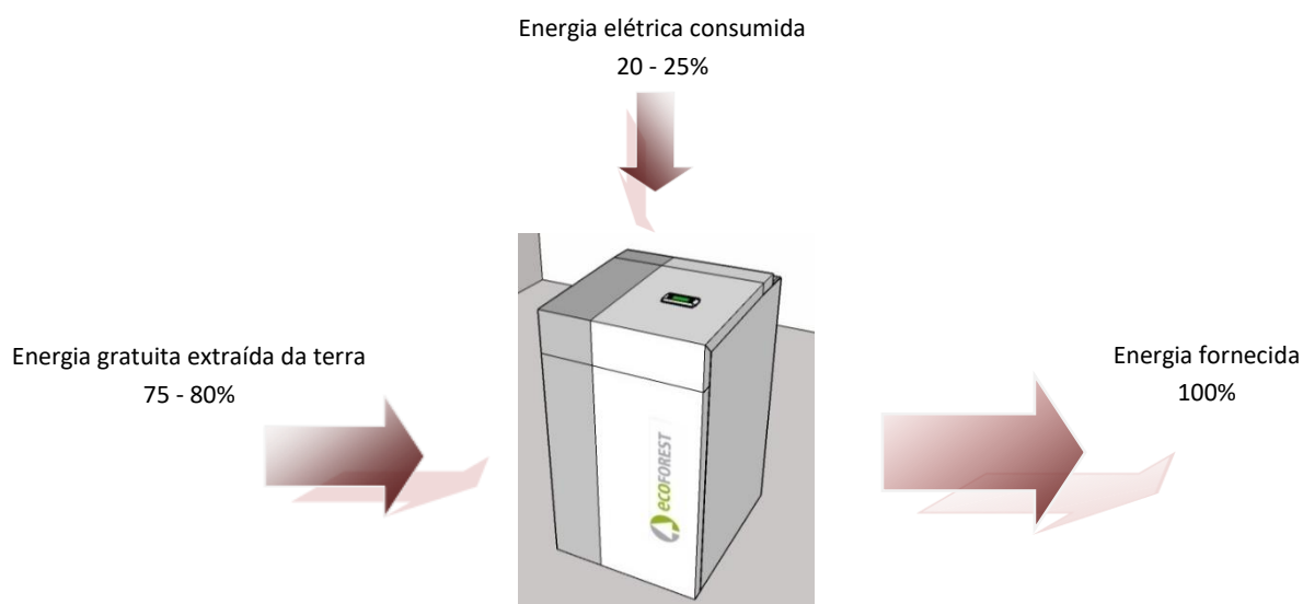
Figura 2.1. Funcionamento de uma bomba de calor geotérmica em condições normais.
