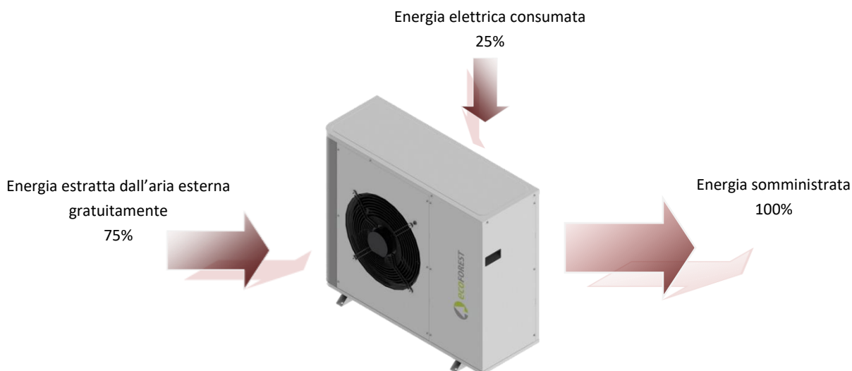
Figura 2.2. Funzionamento di una pompa di calore aerotermica in condizioni normali.
